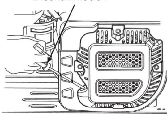
ZAGONSKA ROČICA
