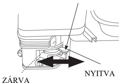
SZÍVÁTOKÁR
