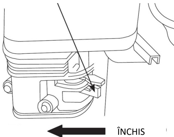
MANETA SUPAPEI COMBUSTIBILULUI
