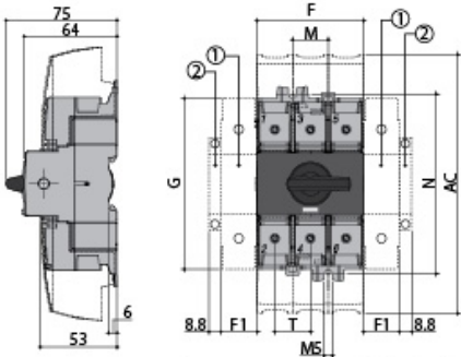
CLBS 100 - CLBS 125 3P
